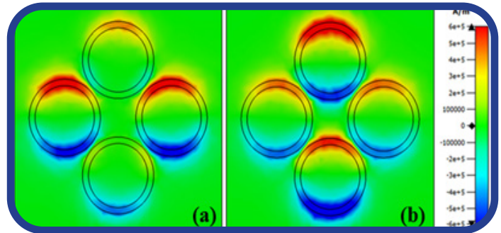
شکل ۵. نمای بالایی توزیع میدان نزدیک شدت میدان مغناطیسی (Hz) در طول موج‌های تشدید (a) \lambda=1151 نانومتر و (b) \lambda=1787 نانومتر.
