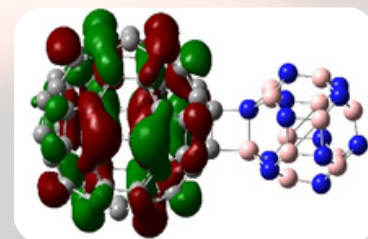
LUMO-D
