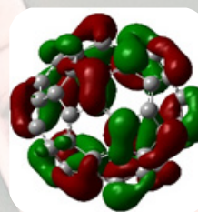
LUMO-c 60
