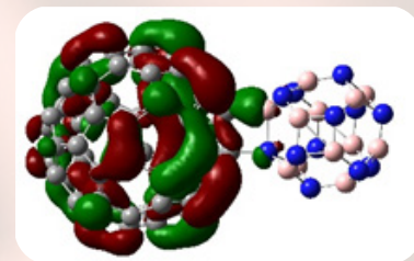
LUMO-C
