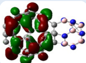
LUMO-A
