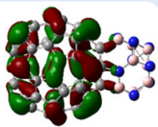
HOMO-A
