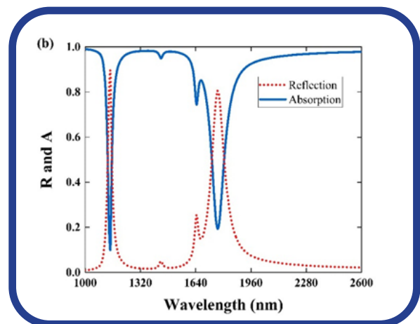
شکل ۲. طیف بازتاب و جذب PRF پیشنهادی (a) با و (b) بدون گرافن تک لایه.
