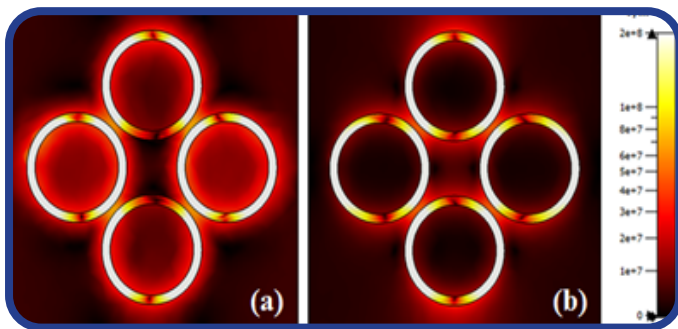
شکل ۳. نمای بالایی از توزیع میدان نزدیک افزایش شدت میدان الکتریکی در طول موج های تشدید (a) \lambda_1 = 1145 نانومتر، و (b) \lambda_2 = 1765 نانومتر.
