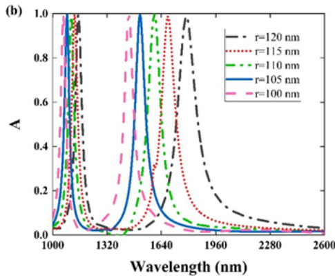
شکل ۶. (a) بازتاب و (b) طیف جذب PRF پیشنهادی برای مقادیر مختلف شعاع شیار استوانه‌ای از r=100\text{ nm} تا r=120\text{ nm} .
