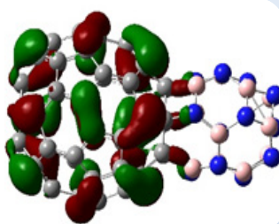
HOMO-B
