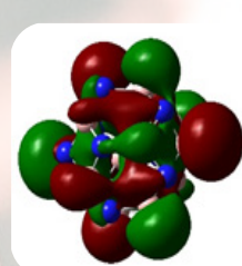
LUMO-B 12 N 12
