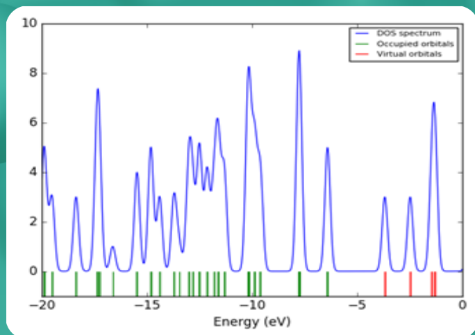
C 60
