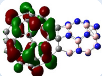
LUMO-B
